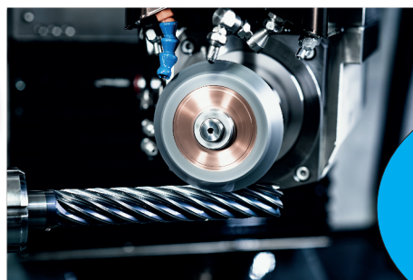
Bearbeitung von Zerspanungs- werkzeugen mit Wunschgeometrie und natürlich auch in Sondermaßen
